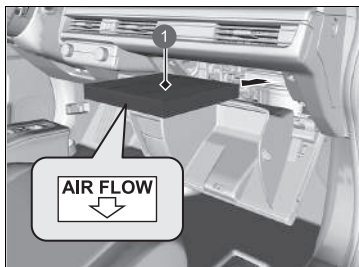
❶ Filtre à poussière et à pollen
