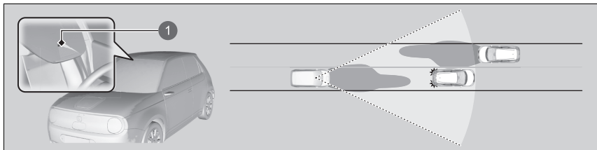
1 Caméra du capteur avant
